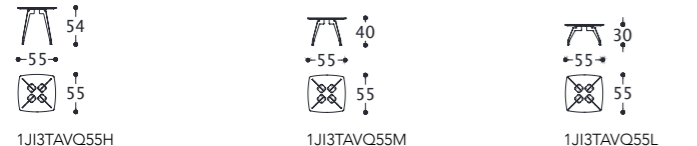
1JI3TAVQ55H
